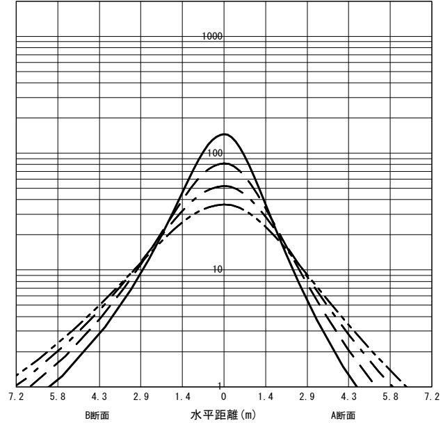
○直射水平面照度 (全光束: 1430 × 1 = 1430lm/台) 照度 (lx) — H1.50m --- H2.00m - - - H2.50m - · - · H3.00m (保守率: 1.00)
