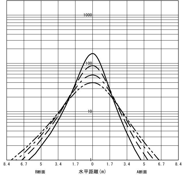
○直射水平面照度 (全光束: 1570 × 1 = 1570lm/台) 照度 (lx) — H1.50m --- H2.00m - - - H2.50m - · - · H3.00m (保守率: 1.00)
