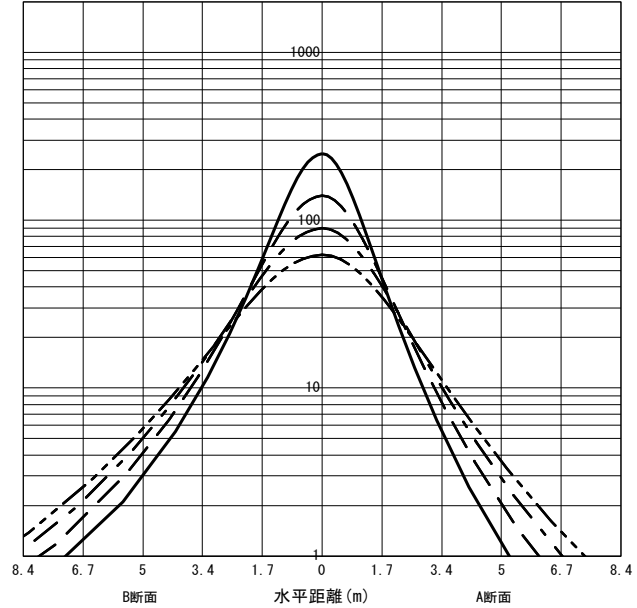
○直射水平面照度 (全光束 : 2440 × 1 = 2440lm/台) 照度 (lx) — H1.50m --- H2.00m - - - H2.50m - · - - H3.00m (保守率 : 1.00)
