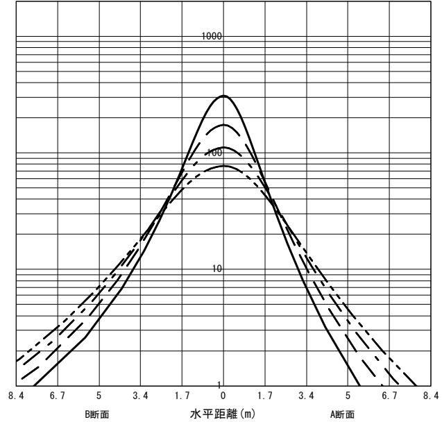
○直射水平面照度 (全光束: 3030 × 1 = 3030lm/台) 照度 (lx) — H1.50m --- H2.00m - - - H2.50m - · - - H3.00m (保守率: 1.00)
