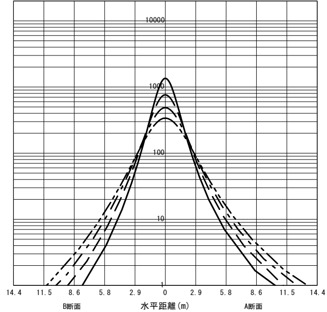
○直射水平面照度 (全光束: 9700 × 1 = 9700lm/台) 照度 (lx) — H1.50m --- H2.00m - - - H2.50m - · - · H3.00m (保守率: 1.00)
