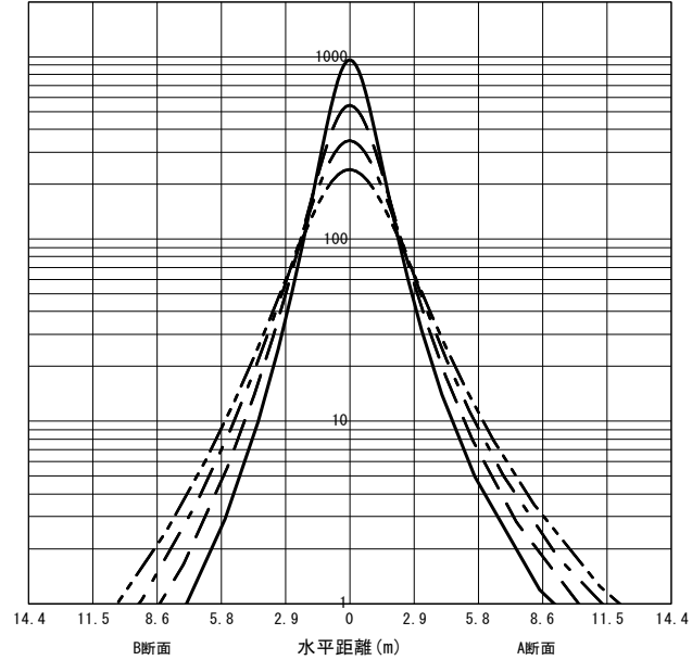
○直射水平面照度 (全光束: 6910 × 1 = 6910lm/台) 照度 (lx) — H1.50m --- H2.00m - - - H2.50m - · - · H3.00m (保守率: 1.00)
