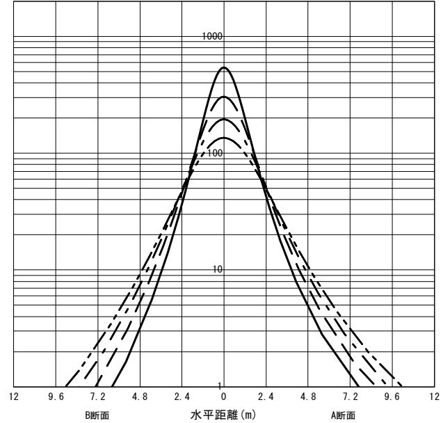
○直射水平面照度 (全光束 : 3890 × 1 = 3890lm/台) 照度 (lx) — H1.50m --- H2.00m - - - H2.50m - · - · H3.00m (保守率 : 1.00)
