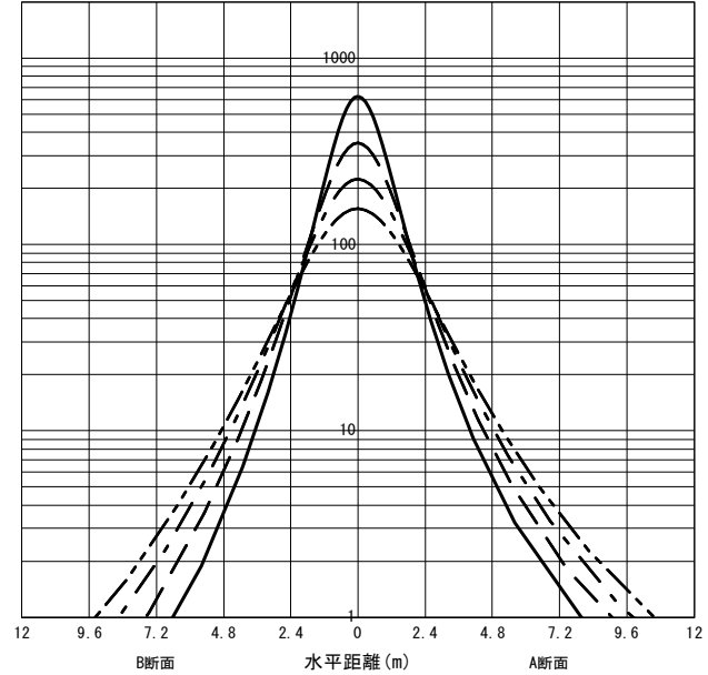
○直射水平面照度 (全光束: 4470 × 1 = 4470lm/台) 照度 (lx) — H1.50m --- H2.00m - - - H2.50m - · - · H3.00m (保守率: 1.00)
