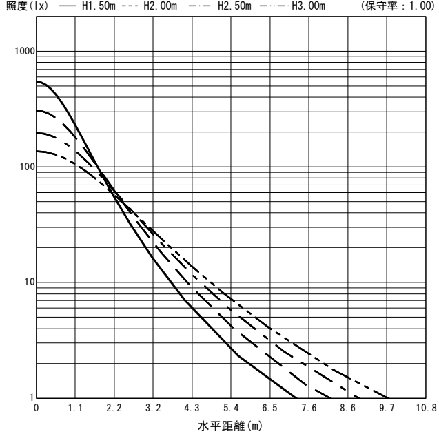
○直射水平面照度 (全光束 : 4000 × 1 = 4000lm/台)
