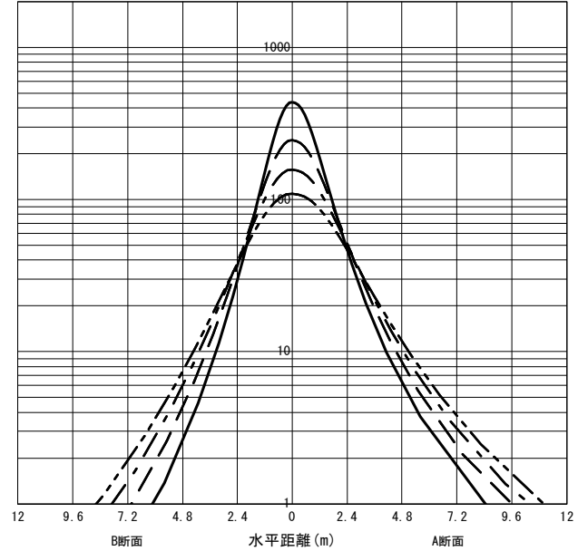
○直射水平面照度 (全光束: 4390 × 1 = 4390lm/台) 照度 (lx) — H1.50m --- H2.00m - - - H2.50m - · - · H3.00m (保守率: 1.00)
