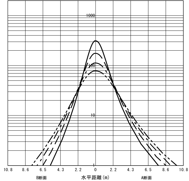
○直射水平面照度 (全光束: 3150 × 1 = 3150lm/台) 照度 (lx) — H1.50m --- H2.00m - - - H2.50m - · - · H3.00m (保守率: 1.00)
