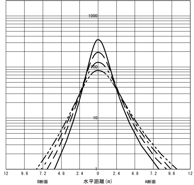
○直射水平面照度 (全光束: 3450 × 1 = 3450lm/台) 照度 (lx) — H1.50m --- H2.00m - - - H2.50m - · - · H3.00m (保守率: 1.00)
