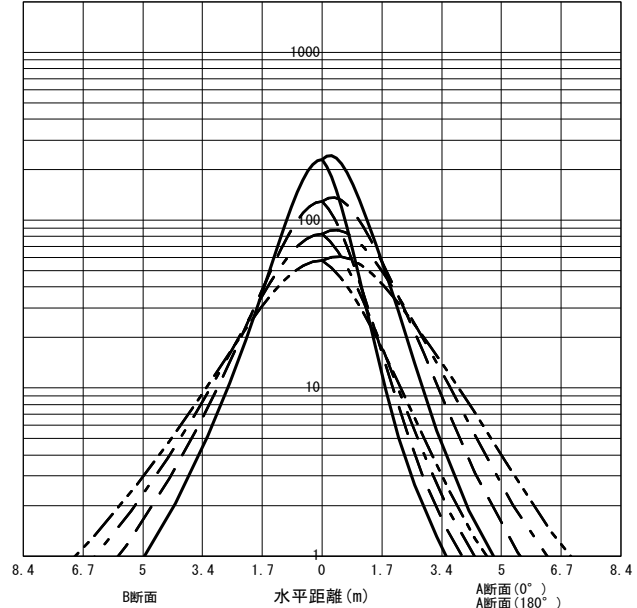
○直射水平面照度 (全光束: 1240 × 1 = 1240lm/台) 照度 (lx) — H1.50m --- H2.00m - - - H2.50m - · - · H3.00m (保守率: 1.00)
