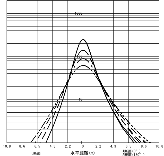
○直射水平面照度 (全光束: 2210 × 1 = 2210lm/台)
