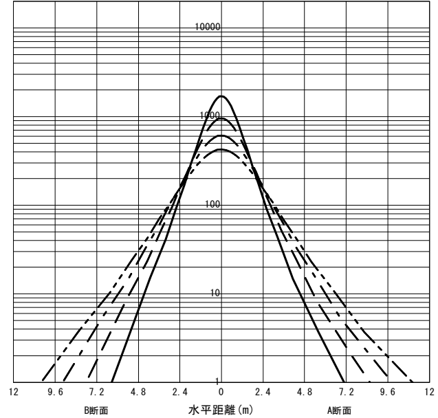
○直射水平面照度 (全光束: 10500 × 1 = 10500lm/台) 照度 (lx) — H1.50m --- H2.00m - - - H2.50m - · - · H3.00m (保守率: 1.00)
