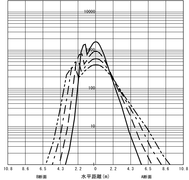
○直射水平面照度 (全光束 : 12900 × 1 = 12900lm/台) 照度 (lx) — H1.50m --- H2.00m - - - H2.50m - · - · H3.00m (保守率 : 1.00)
