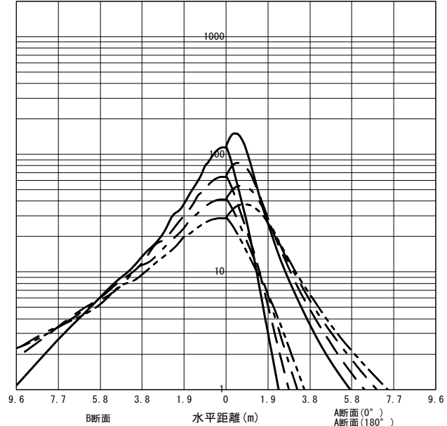
○直射水平面照度 (全光束: 1400 × 1 = 1400lm/台) 照度 (lx) — H1.50m --- H2.00m - - - H2.50m - · - · H3.00m (保守率: 1.00)
