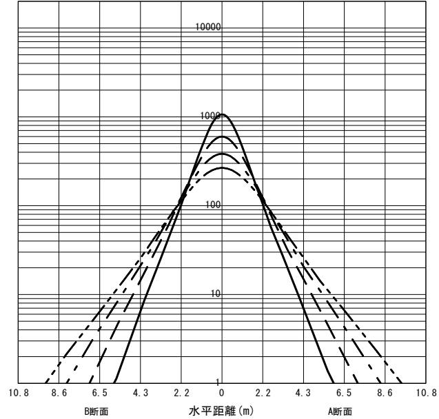
○直射水平面照度 (全光束: 6500 × 1 = 6500lm/台) 照度 (lx) — H1.50m --- H2.00m - - - H2.50m - · - · H3.00m (保守率: 1.00)
