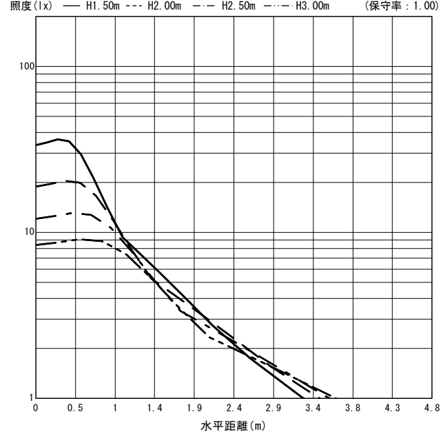
○直射水平面照度 (全光束: 440 × 1 = 440lm/台)
