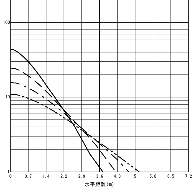
○直射水平面照度 (全光束：480 × 1 = 480lm/台)
