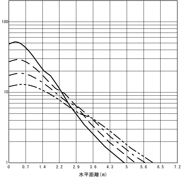
○直射水平面照度 (全光束 : 920 × 3 = 2760lm/台)
