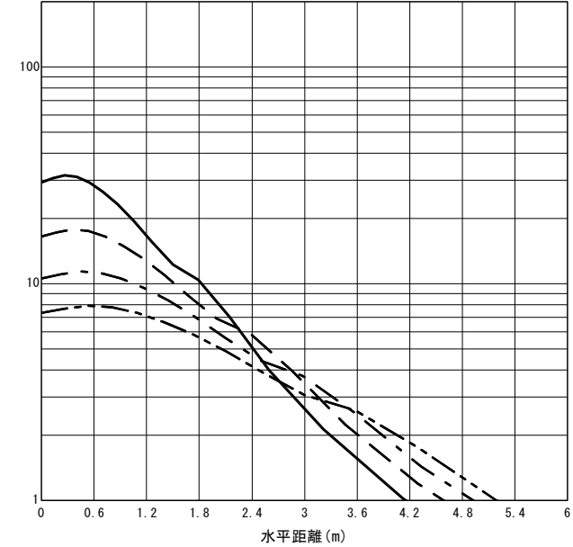
○直射水平面照度 (全光束 : 560 × 3 = 1680lm/台) 照度 (lx) — H1.50m --- H2.00m - - - H2.50m - · - · H3.00m (保守率 : 1.00)
