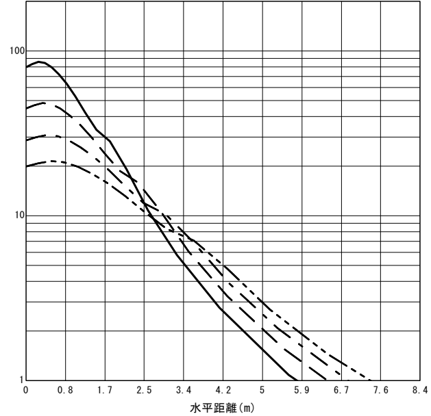
○直射水平面照度 (全光束 : 760 × 6 = 4560lm/台) 照度 (lx) — H1.50m --- H2.00m - - - H2.50m - · - · H3.00m (保守率 : 1.00)
