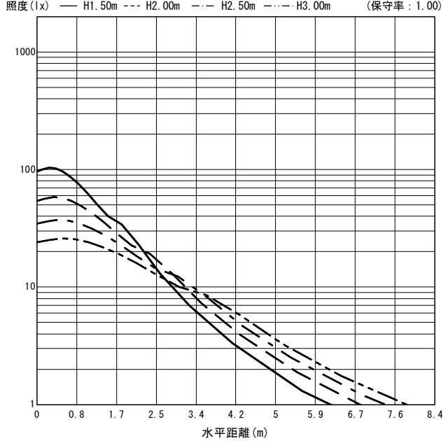
○直射水平面照度 (全光束 : 920 × 6 = 5520lm/台)
