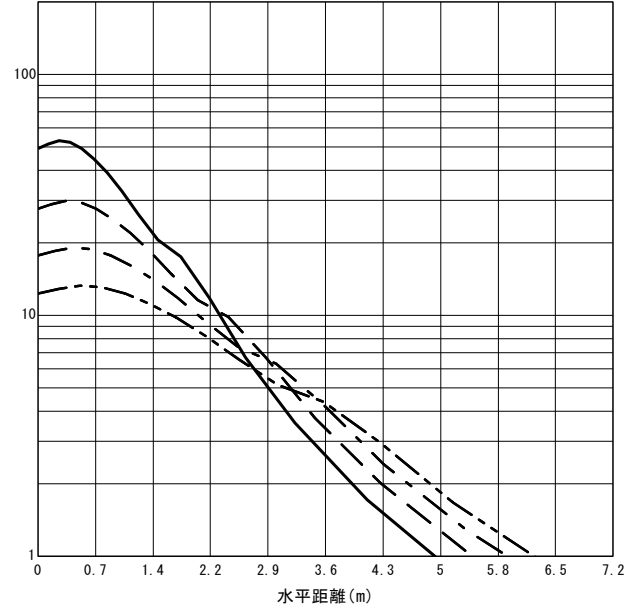
○直射水平面照度 (全光束 : 470 × 6 = 2820lm/台) 照度 (lx) — H1.50m --- H2.00m - - - H2.50m - · - · H3.00m (保守率 : 1.00)
