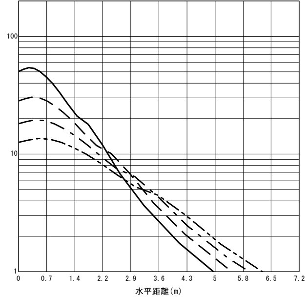
○直射水平面照度 (全光束 : 480 × 6 = 2880lm/台) 照度 (lx) — H1.50m --- H2.00m - - - H2.50m - · - · H3.00m (保守率 : 1.00)
