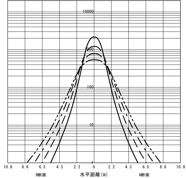
○直射水平面照度 (全光束 : 10000 × 1 = 10000lm/台) 照度 (lx) — H1.50m --- H2.00m - - - H2.50m - · - · - H3.00m (保守率 : 1.00)
