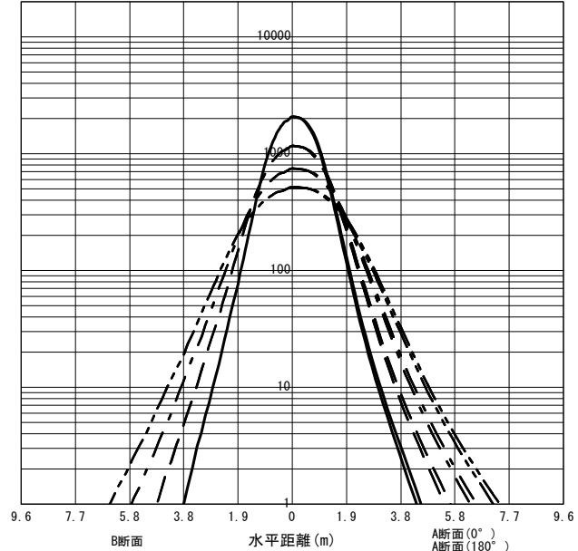
○直射水平面照度 (全光束: 7800 × 1 = 7800lm/台) 照度 (lx) — H1.50m --- H2.00m - - - H2.50m - · - · H3.00m (保守率: 1.00)
