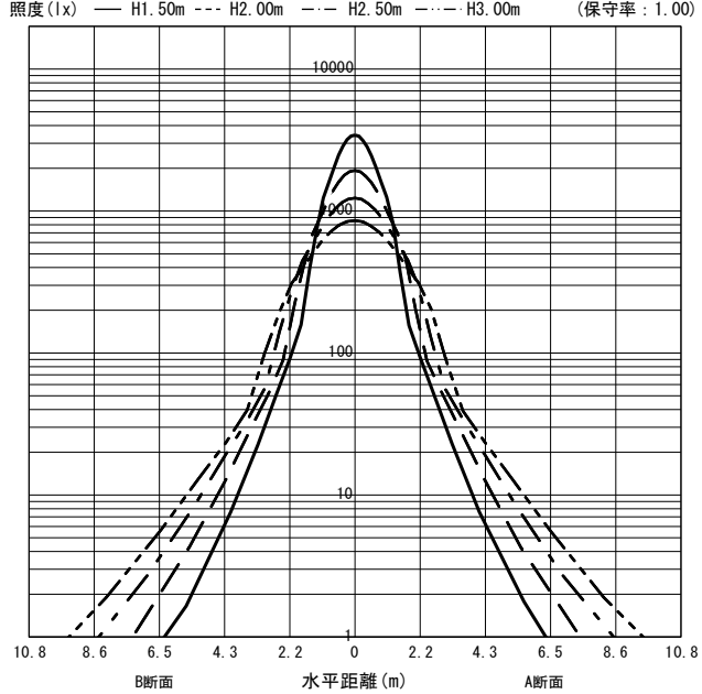
○直射水平面照度 (全光束 : 12500 × 1 = 12500lm/台)
