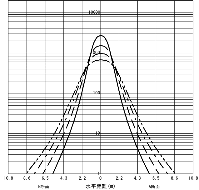
○直射水平面照度 (全光束 : 12500 × 1 = 12500lm/台) 照度 (lx) — H1.50m --- H2.00m - - - H2.50m - · - - H3.00m (保守率 : 1.00)
