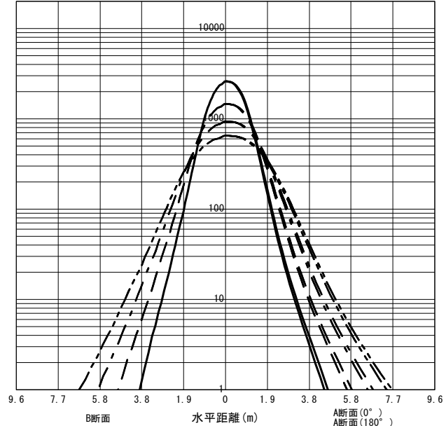
○直射水平面照度 (全光束: 9800 × 1 = 9800lm/台) 照度 (lx) — H1.50m --- H2.00m - - - H2.50m - · - · H3.00m (保守率: 1.00)
