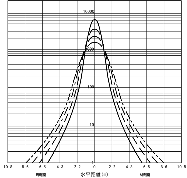
○直射水平面照度 (全光束 : 15300 × 1 = 15300lm/台) 照度 (lx) — H1.50m --- H2.00m - - - H2.50m - · - · H3.00m (保守率 : 1.00)
