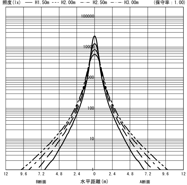
○直射水平面照度 (全光束 : 20300 × 1 = 20300lm/台)
