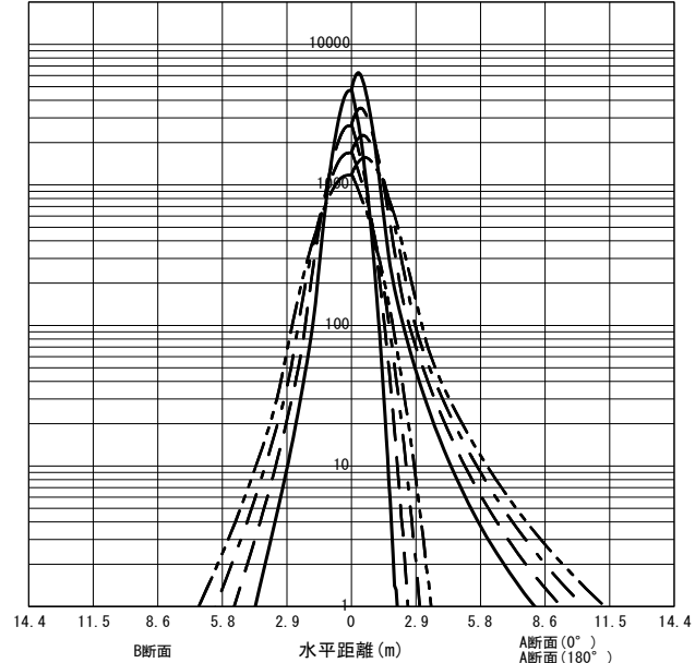
○直射水平面照度 (全光束: 12000 × 1 = 12000lm/台) 照度 (lx) — H1.50m --- H2.00m - - - H2.50m - · - · H3.00m (保守率: 1.00)
