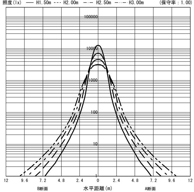
○直射水平面照度 (全光束 : 31200 × 1 = 31200lm/台)
