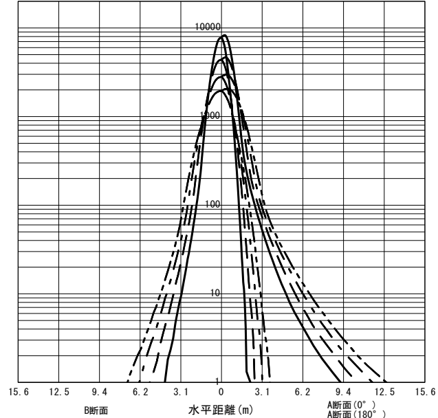
○直射水平面照度 (全光束 : 18000 × 1 = 18000lm/台) 照度 (lx) — H1.50m --- H2.00m - - - H2.50m - · - · - H3.00m (保守率 : 1.00)
