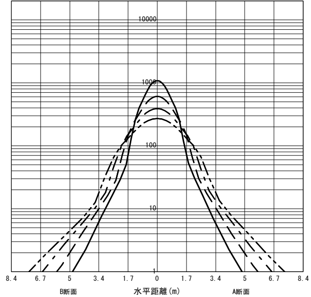
○直射水平面照度 (全光束: 4000 × 1 = 4000lm/台) 照度 (lx) — H1.50m --- H2.00m - - - H2.50m - · - · H3.00m (保守率: 1.00)
