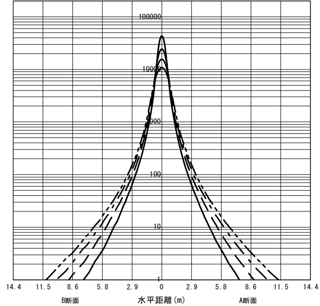
○直射水平面照度 (全光束 : 39200 × 1 = 39200lm/台) 照度 (lx) — H1.50m --- H2.00m - - - H2.50m - · - · H3.00m (保守率 : 1.00)
