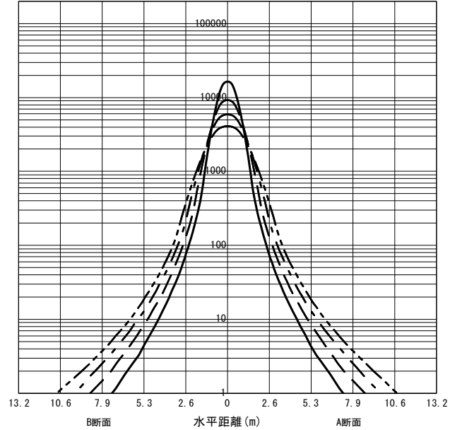
○直射水平面照度 (全光束: 40100 × 1 = 40100lm/台) 照度 (lx) — H1.50m --- H2.00m - - - H2.50m - · - · H3.00m (保守率: 1.00)
