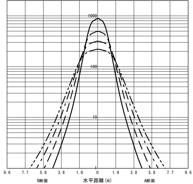
○直射水平面照度 (全光束: 4400 × 1 = 4400lm/台) 照度 (lx) — H1.50m --- H2.00m - - - H2.50m - · - · H3.00m (保守率: 1.00)
