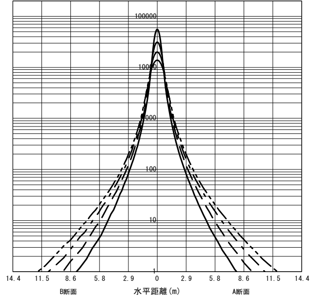
○直射水平面照度 (全光束 : 50200 × 1 = 50200lm/台) 照度 (lx) — H1.50m --- H2.00m - - - H2.50m - · - · H3.00m (保守率 : 1.00)
