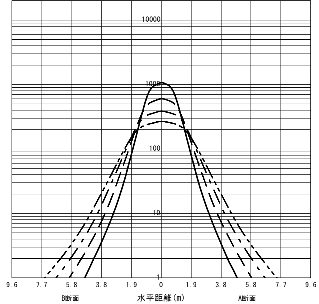
○直射水平面照度 (全光束: 5300 × 1 = 5300lm/台) 照度 (lx) — H1.50m --- H2.00m - - - H2.50m - · - · H3.00m (保守率: 1.00)
