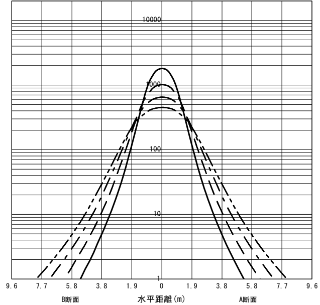
○直射水平面照度 (全光束: 8000 × 1 = 8000lm/台) 照度 (lx) — H1.50m --- H2.00m - - - H2.50m - · - · H3.00m (保守率: 1.00)
