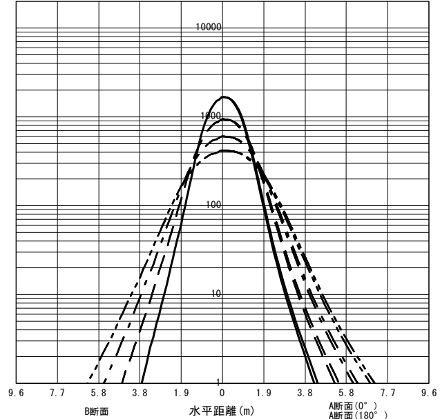
○直射水平面照度 (全光束: 6300 × 1 = 6300lm/台) 照度 (lx) — H1.50m --- H2.00m - - - H2.50m - · - · H3.00m (保守率: 1.00)
