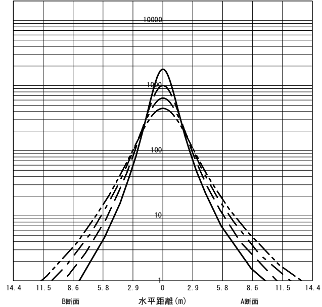
○直射水平面照度 (全光束 : 10980 × 1 = 10980lm/台) 照度 (lx) — H1.50m --- H2.00m - - - H2.50m - · - · H3.00m (保守率 : 1.00)
