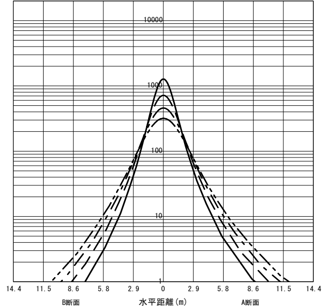
○直射水平面照度 (全光束: 7820 × 1 = 7820lm/台) 照度 (lx) — H1.50m --- H2.00m - - - H2.50m - · - · H3.00m (保守率: 1.00)
