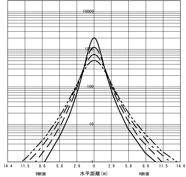
○直射水平面照度 (全光束 : 12420 × 1 = 12420lm/台) 照度 (lx) — H1.50m --- H2.00m - - - H2.50m - · - · - H3.00m (保守率 : 1.00)
