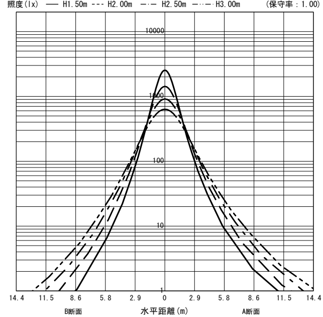
○直射水平面照度 (全光束 : 15540 × 1 = 15540lm/台)
