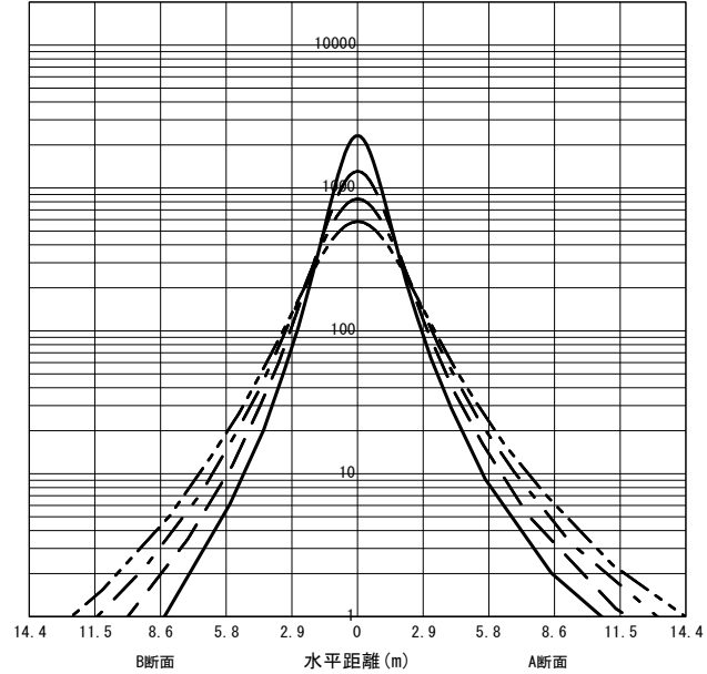
○直射水平面照度 (全光束 : 14280 × 1 = 14280lm/台) 照度 (lx) — H1.50m --- H2.00m - - - H2.50m - · - · H3.00m (保守率 : 1.00)
