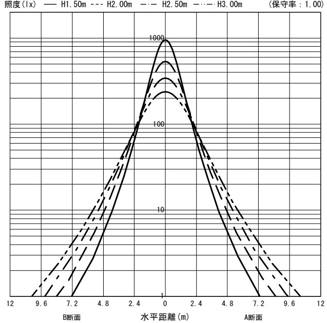
○直射水平面照度 (全光束: 5940 × 1 = 5940lm/台)
